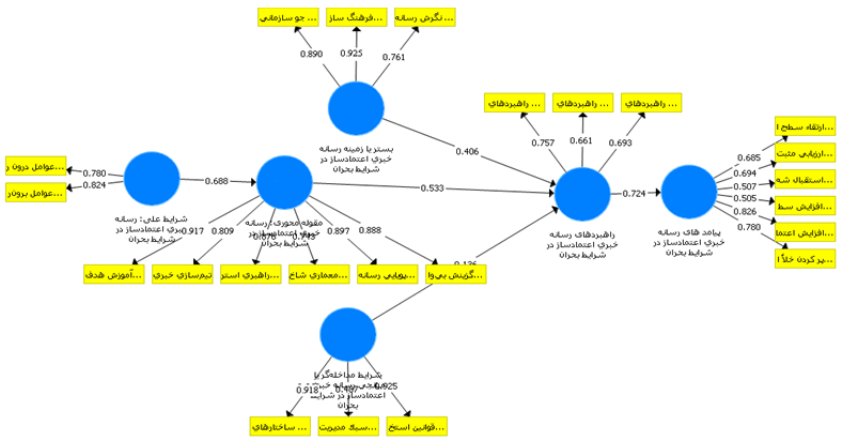
شکل ۳. مدل انعکاسی پژوهش در حالت تخمین ضرایب استاندارد
