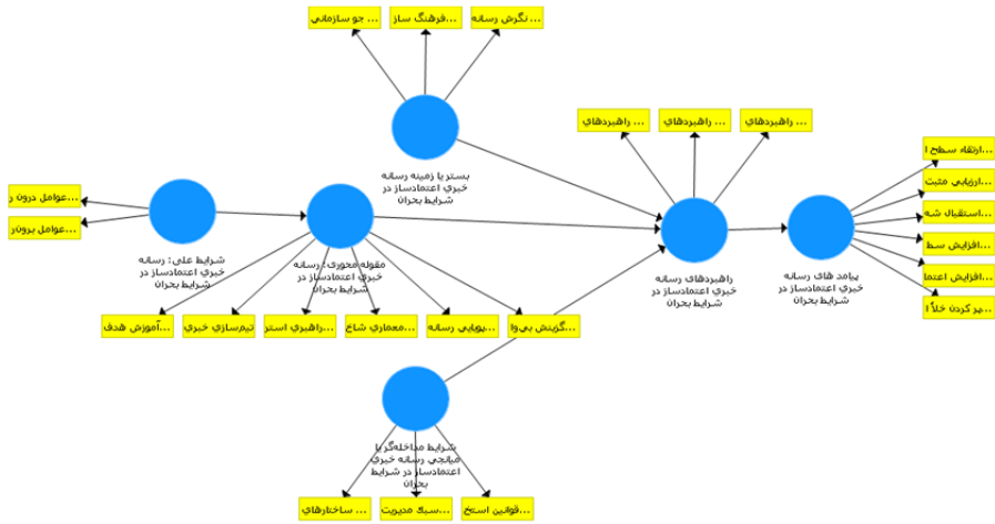
شکل ۲. مدل ساختاری پژوهش
