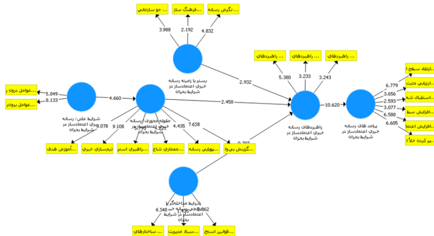
شکل شماره ۴. مدل انعکاسی پژوهش در حالت معناداری ضرایب
